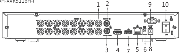
DH-XVR5116H-I
